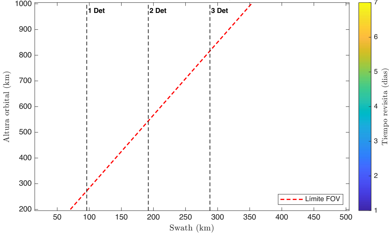
Tiempo Revisita - 1 Satelite(s); 2 Telescopio(s): Refractivo; Detector 1 (Blanco: \geq 7 dias)
